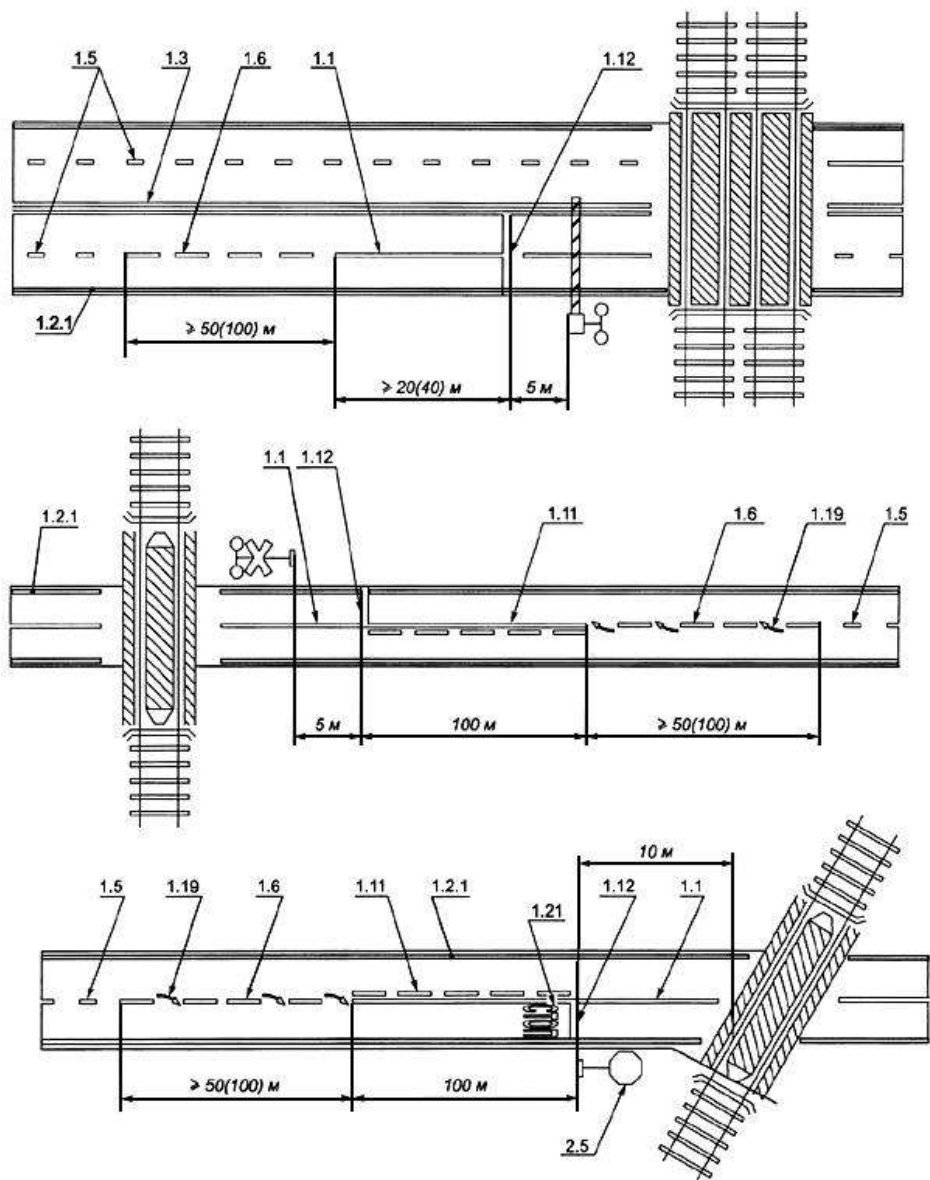
Рисунок В.17 - Примеры разметки участка дороги на подъезде к железнодорожному проезду
